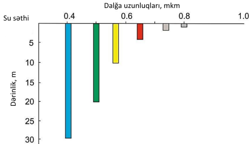
Şəkil 5. Günəş işığının su sütununa təsir etmə dərinliyi [8]
