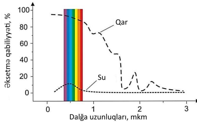
Şəkil 1. Su və qarın əksətmə qabiliyyəti [6]
