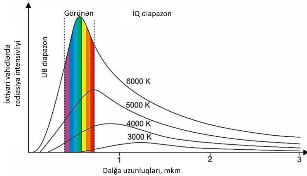
Şəkil 3. Temperaturdan asılı olaraq tamamilə qara bir cismin şüalanma intensivliyinin dəyişməsi [8]
