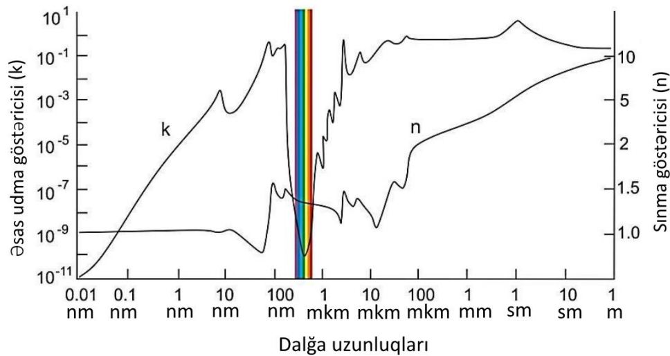
Şəkil 2. Geniş spektrdə təmiz suyun optik sabitləri [8]
