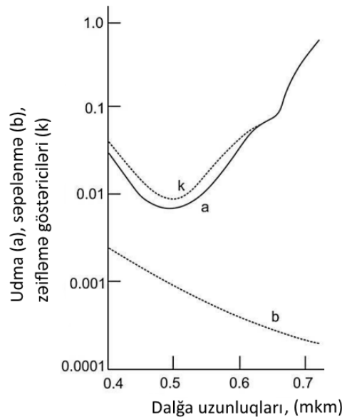
Şəkil 4. Spektrin görünən hissəsində təmiz suyun udulması, dağılması və zəifləməsi göstəriciləri [8]
