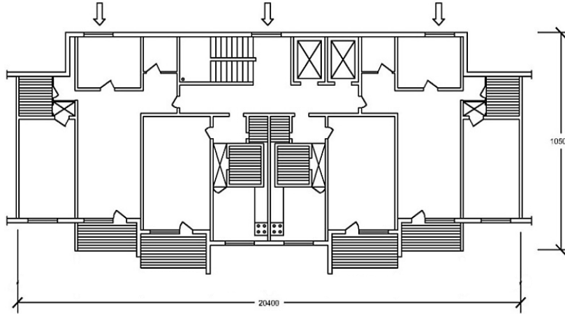
Şəkil 3. Yüksək səs-izolyasiyalı ekran yaşayış evinin planı [5]
