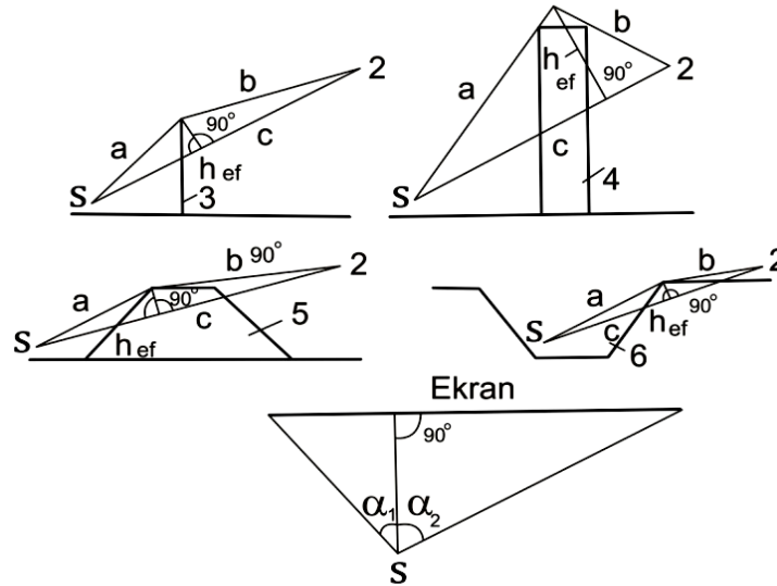
Şəkil 5. Ekran hesabına səsin azalmasını təyin etmək üçün hesablama sxemi.
