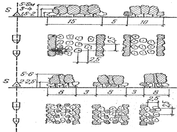
Şəkil 4. Səs-küy mənbəyinə görə müxtəlif formada salınmış yaşıllıq zolaqları [5]
