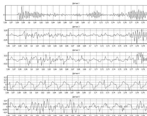
Şəkil 5. Binaanın mərtəbələri boyunca sərbəst rəqslər. X oxu üzrə rəqslər. fayl: asinaq1x1x [4]
