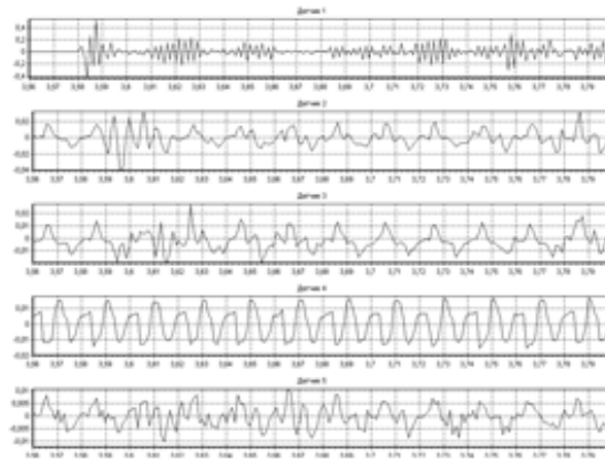
Şəkil 4. Binaanın mərtəbələri boyunca sərbəst rəqslər. Y oxu üzrə rəqslər. fayl: asinaq1x1y [4]
