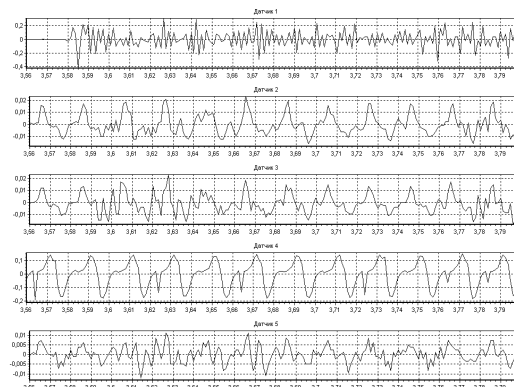
Şəkil 5. Binaanın mərtəbələri boyunca sərbəst rəqslər. X oxu üzrə rəqslər. fayl: asinaq1x1x [4]
