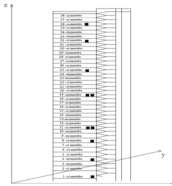
Şəkil 3. Sınaq zamanı seysmoqəbuledicilərin binada yerləşmə səviyyələri [3]
