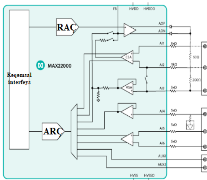
Şəkil 3. MAX22000 ilə konfigurasiya edilən Analıq modul [6]
