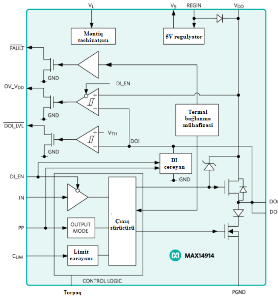
Şəkil 5. MAX14914 ilə rəqəmsal giriş və çıxışın konfigurasiyası [6]
