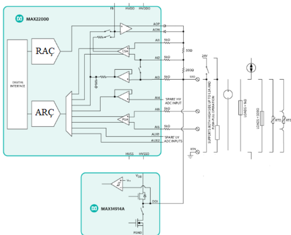
Şəkil 2. Konfigurasiya edilən MAX22000 [4]
