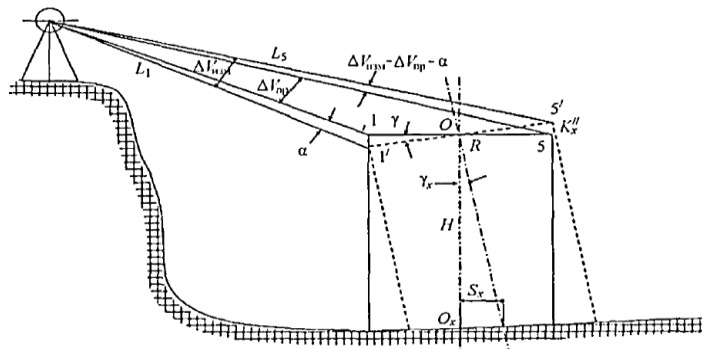
Şəkil 2. Bir stansiyadan silindrik qabıqın rulonunun təyini [2]
