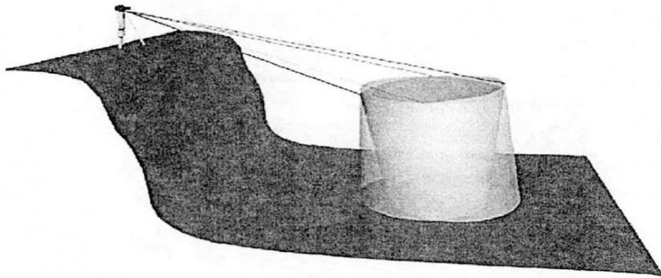
Şəkil 3. Rulonun təyini metodunun üçölçülü modeli [3]
