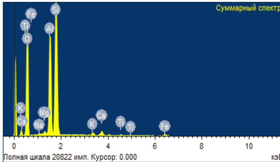
Şəkil 2. Aşağı Güzdək gili, şamot və uçucu kül tərkibli keramik materialın mikrozonnd analizi [5]
