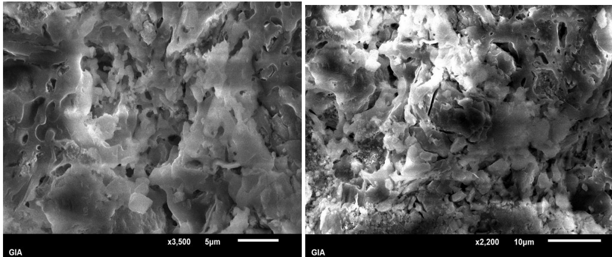
Şəkil 3. Aşağı Güzdək gili, şamot və uçucu kül tərkibli keramik materialın mikroşəkilləri [5]
