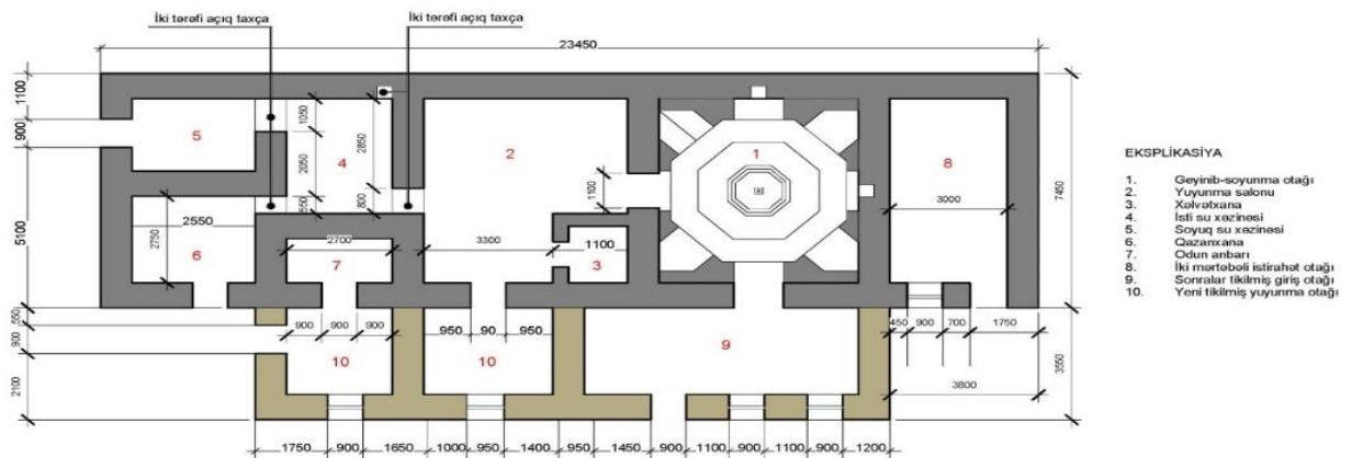
Şəkil 4. Gülablı kəndi ərazisində yerləşən hamamın planı (XIX əsr)
